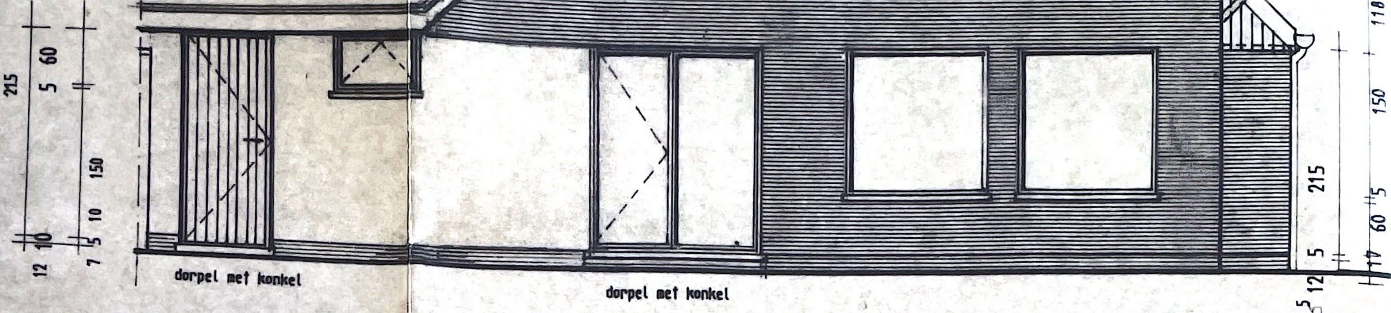
ACHTERGEVEL 1/50
