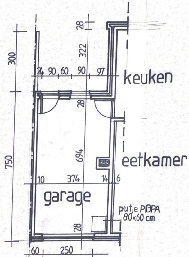
GRONDPLAN TYPE 1 D b 3/6 type met zuidoerijentatie voorzijde.
