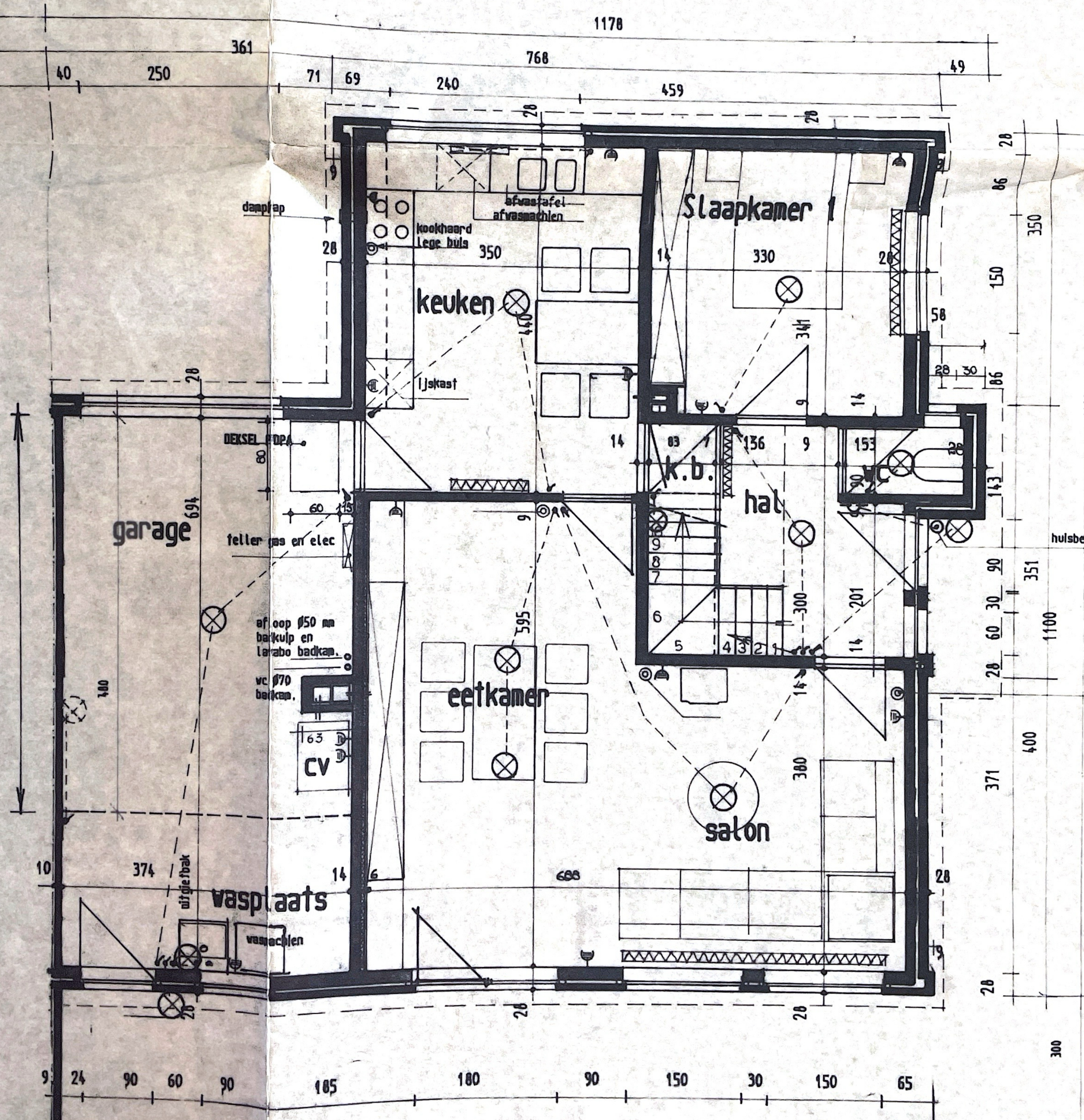
PLAN GELIJKVLOERS 1/50
